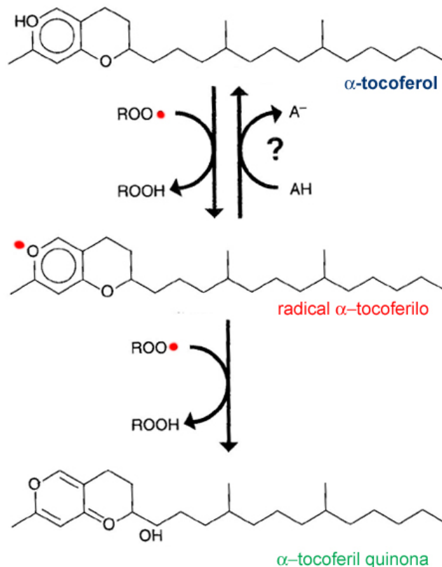
Figura 3. Efecto antioxidante del \alpha -tocoferol ( http://www.iqb.es/cbasicas/farma/farma04/t001.htm ).
