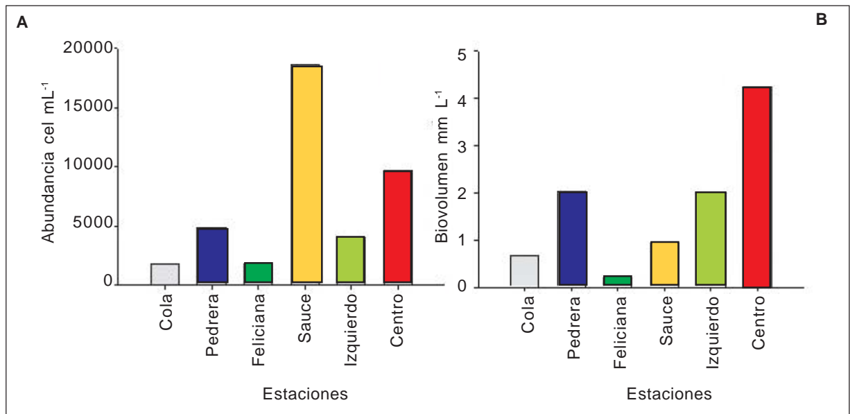
Figura 6. A: abundancia promedio y B: biovolumen promedio de fitoplancton de todo el periodo de estudio.
