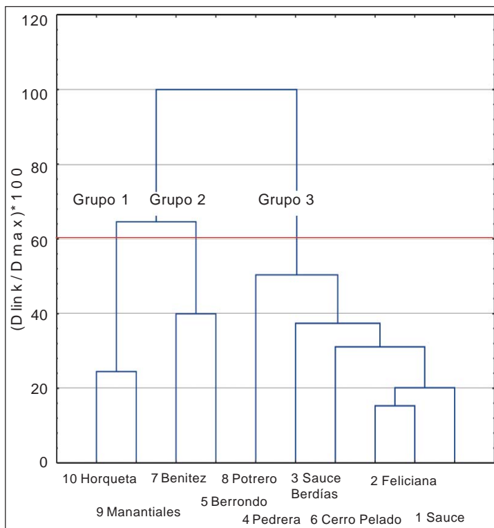
Figura 3. Agrupamiento de las cuencas según los parámetros físico-químicos de sus arroyos.
