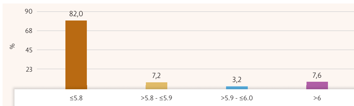
Figura 12. Distribución (%) de pH para el total de las canales evaluadas.
