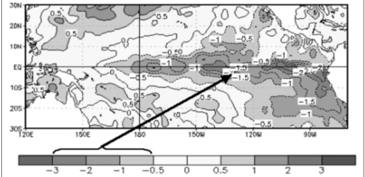
Figura 2 Anomalías de Temperatura del Océano Pacífico. Fuente: NCEP - NOAA
