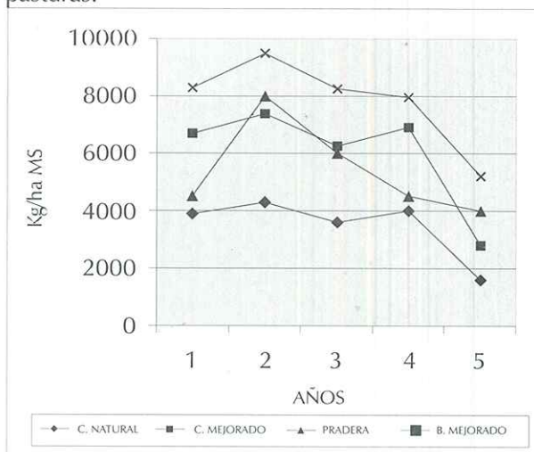
Figura 2. Producción de Forraje anual de distintas pasturas.
