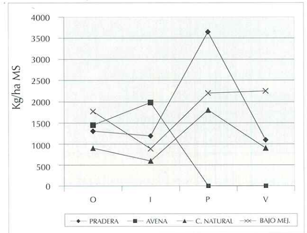
Figura 3. Producción estacional de distintas alternativas forrajeras.
