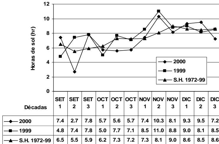
Figura 2.3. Evolución de las horas de sol por década desde Setiembre a Diciembre para la zafra 2000/01, 1999/00 y la serie histórica (1972-99).
