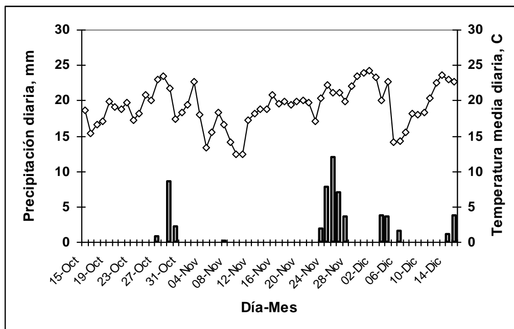
Figura. 7.1- Precipitación y temperatura media diaria en el período del 15 de octubre al 15 de diciembre de 2000. Paso de la Laguna. Treinta y Tres.
