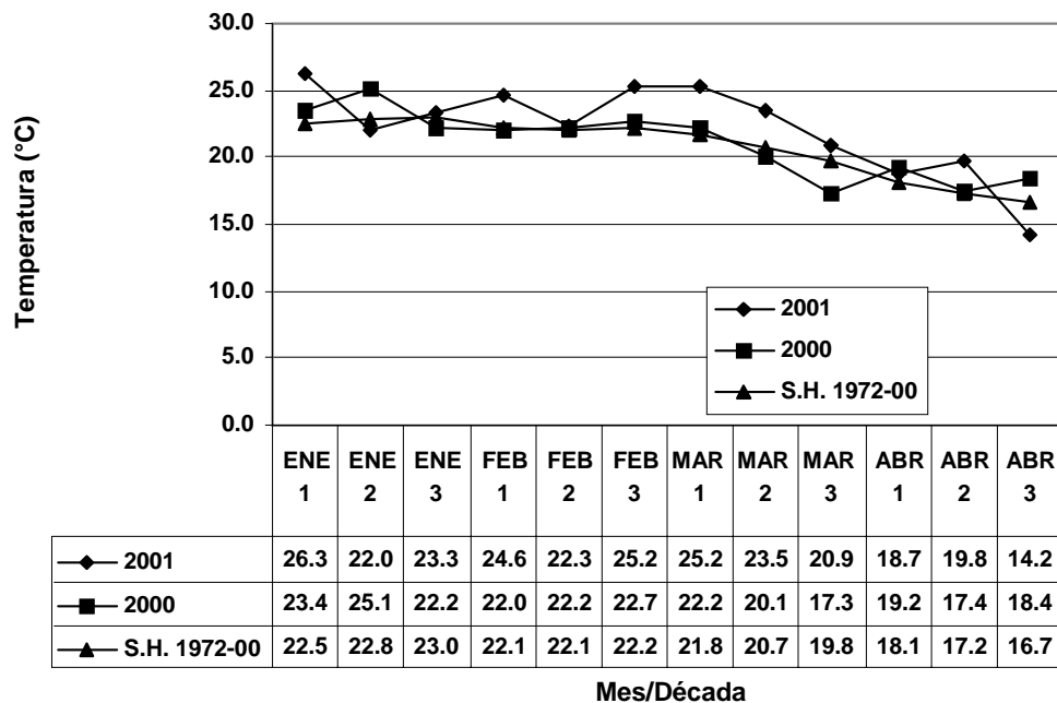
Figura 2.6. Evolución de la temperatura media del aire por década desde Enero a Abril para la zafra 2000/01, 1999/00 y la serie histórica (1972-2000).
