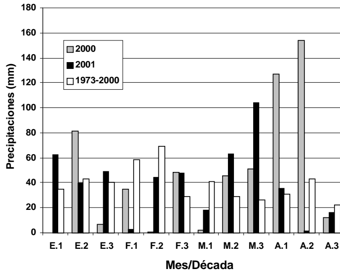
Figura 2.2 Precipitaciones por década desde enero a abril en la zafra anterior (1999/00), 2000/01 y promedio de la serie histórica 1973-2000.
