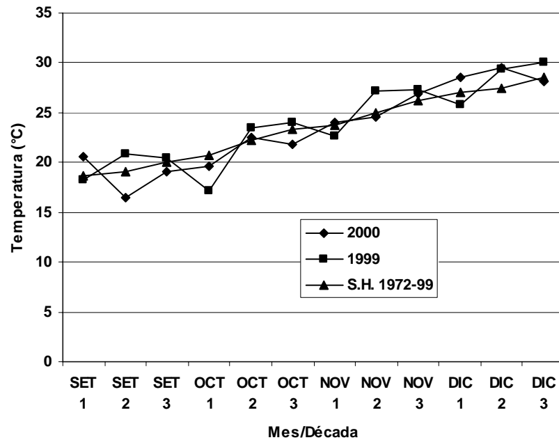
Figura 2.7. Evolución de la temperatura máxima del aire por década desde Setiembre a Diciembre para la zafra 2000/01, 1999/00 y la serie histórica (1972-99).
