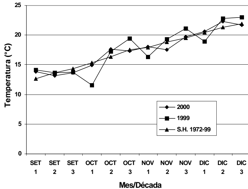
Figura 2.5. Evolución de la temperatura media del aire por década desde Setiembre a Diciembre para la zafra 2000/01, 1999/00 y la serie histórica (1972-99).
