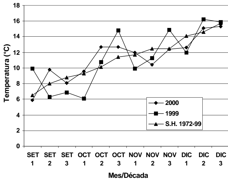
Figura 2.9. Evolución de la temperatura mínima del aire por década desde Setiembre a Diciembre para la zafra 2000/01, 1999/00 y la serie histórica (1972-99).
