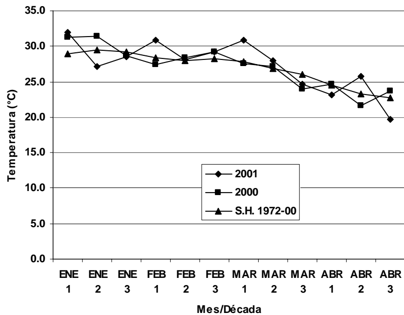
Figura 2.8. Evolución de la temperatura máxima del aire por década desde Enero a Abril para la zafra 2000/01, 1999/00 y la serie histórica (1972-2000).
