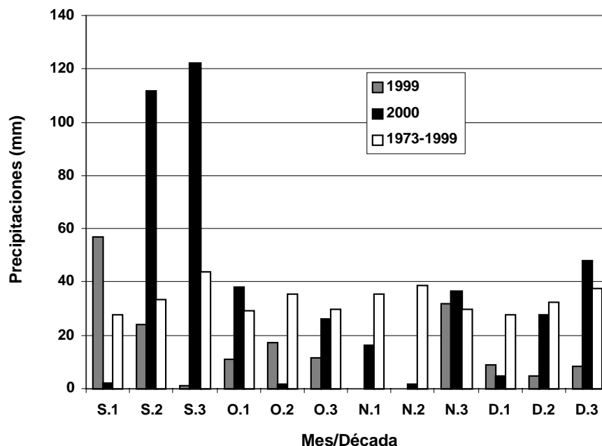
Figura 2.1 Precipitaciones por década desde Setiembre a Diciembre en la zafra anterior (1999/00), 2000/01 y promedio de la serie histórica 1973-99.
