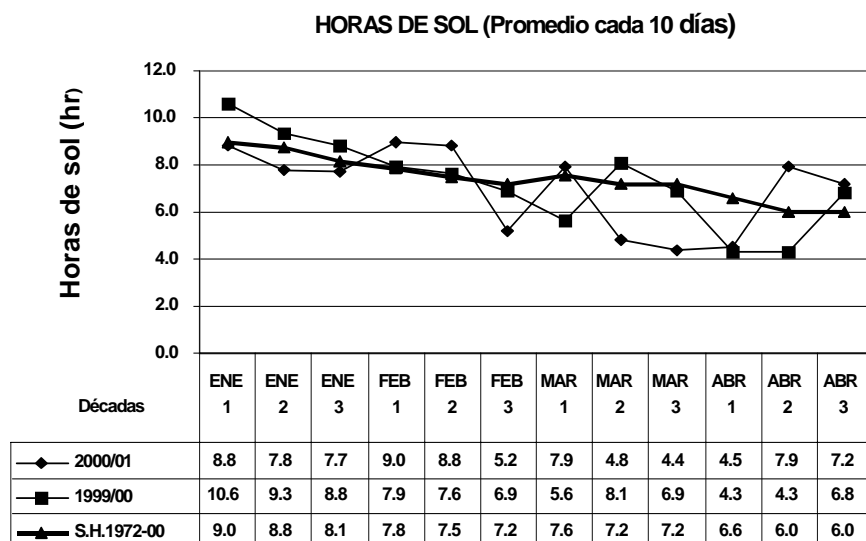
Figura 2.4. Evolución de las horas de sol por década desde Enero a Abril para la zafra 2000/01, 1999/00 y la serie histórica (1972-2000).
